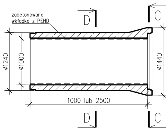
PRZEKRÓJ E-E
